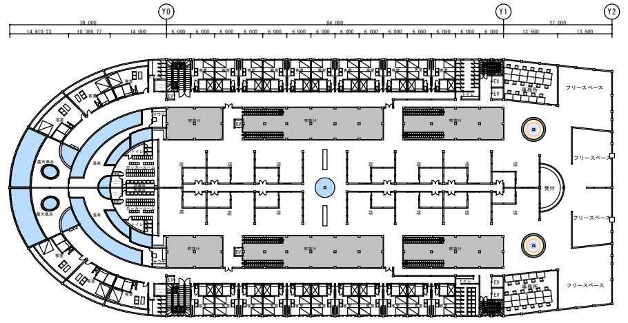
8階 平面図 1/650
