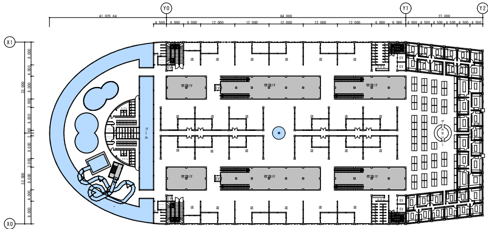
7階 平面図 1/650
