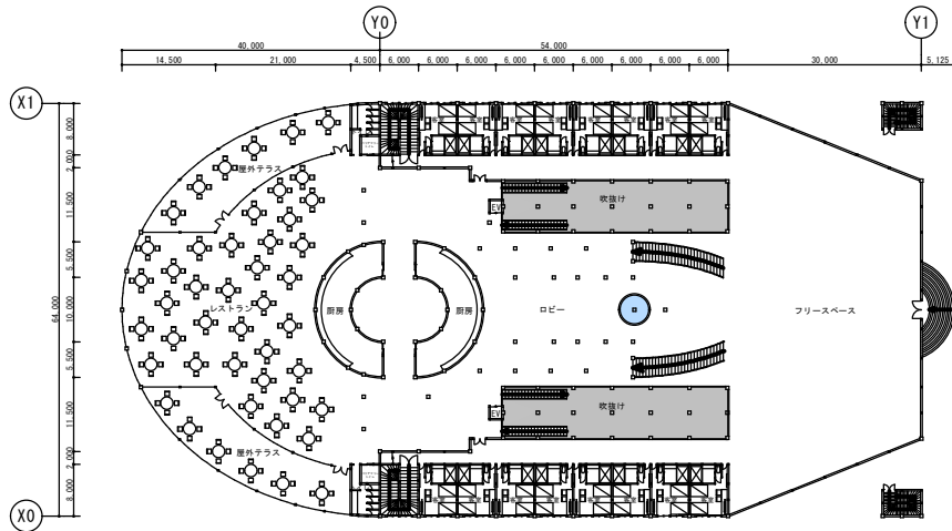
11階 平面図 1/650
