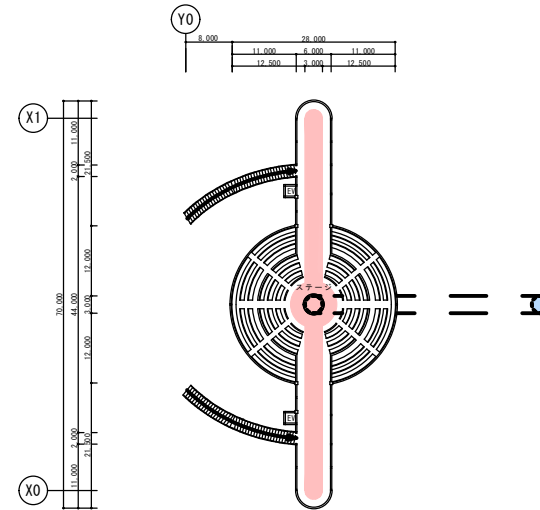
13階 平面図 1/650
