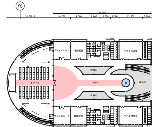
12階 平面図 1/650
