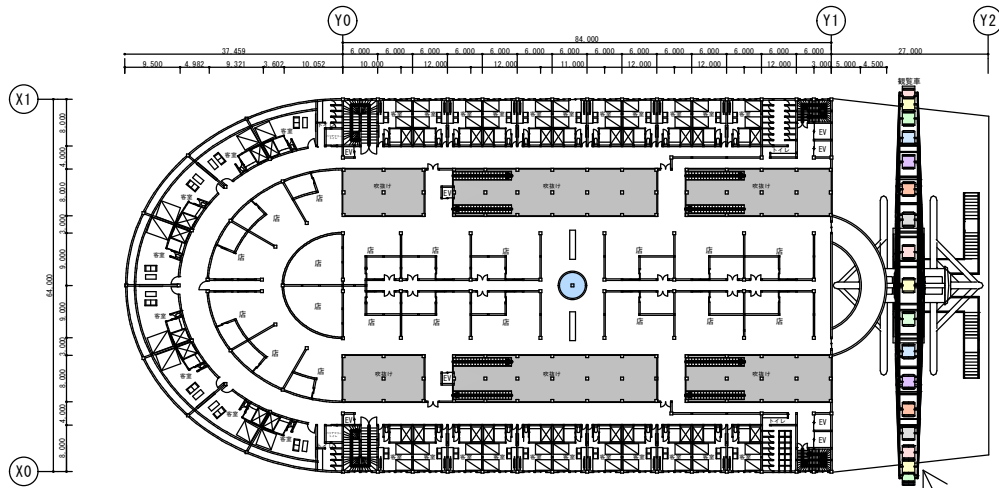
10階 平面図 1/650
